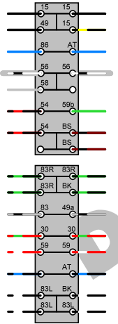
Klemmleiste A SR50
